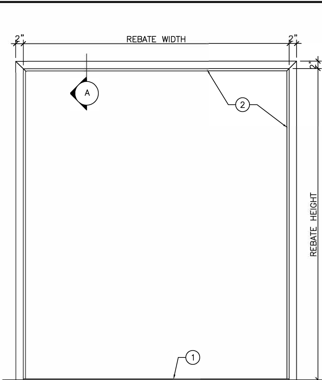
ELEVATION \frac{3}{4}'' = 1'-0''
