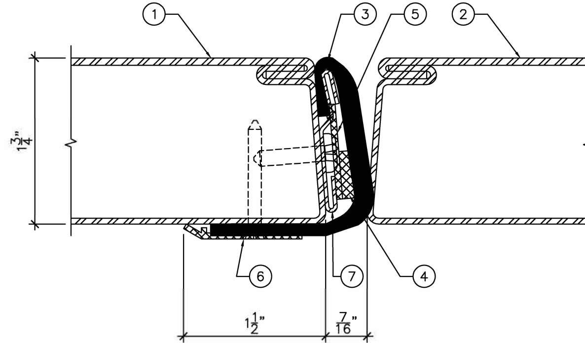
ASTRAGAL SECTION 1'-0" = 1'-0"
