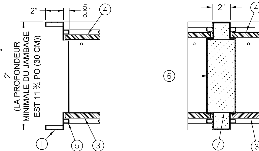
COUPE A-A
