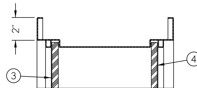
COUPE D-D
