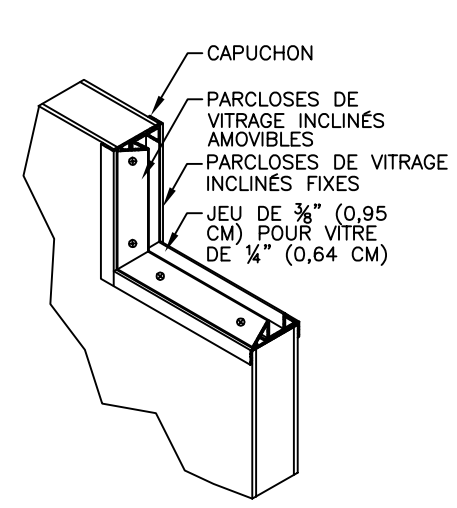
ENSEMBLE SPÉCIAL EN BISEAU POUR VITRAGE
