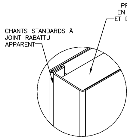
CHANT À JOINT RABATTU STANDARD ET DÉTAIL DE PROFILÉ STANDARD
