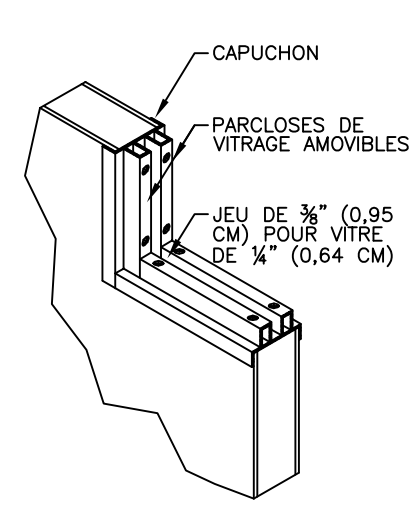
ENSEMBLE POUR VITRAGE STANDARD
