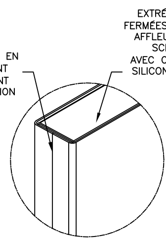
CHANT SANS JOINT APPARENT EN OPTION ET DÉTAIL DE CAPUCHON AFFLEURANT
