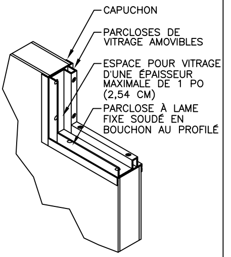
ENSEMBLE POUR VITRAGE ÉPAIS
