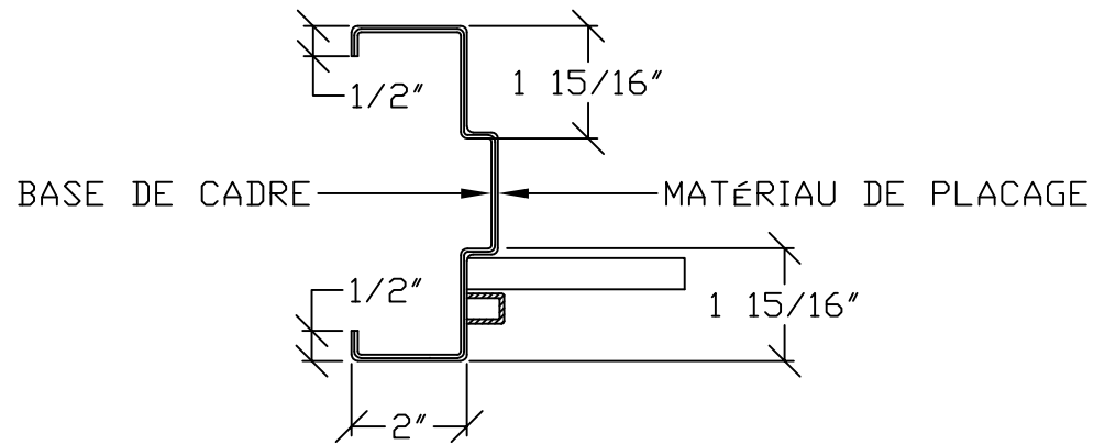
COUPE A - CADRE PLAQUÉ TYPE
