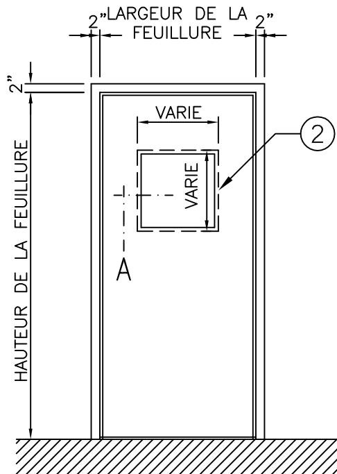
ÉLÉVATION
