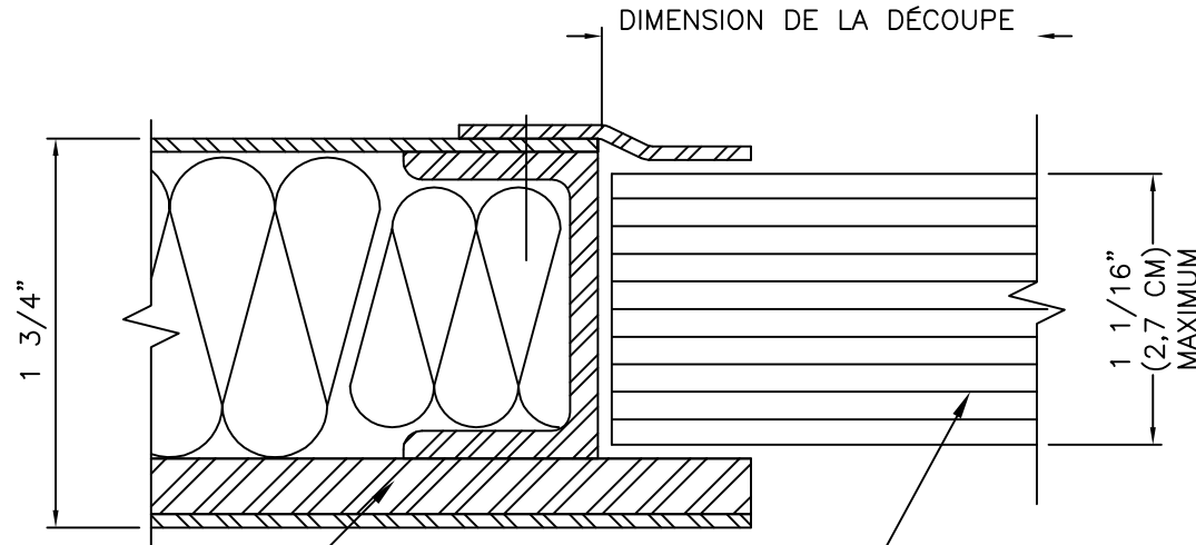
COUPE 'A'
