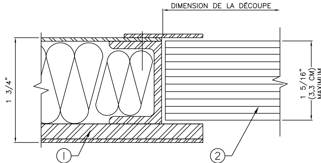
COUPE 'A'
