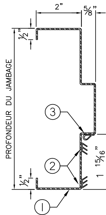
COUPE A-A
