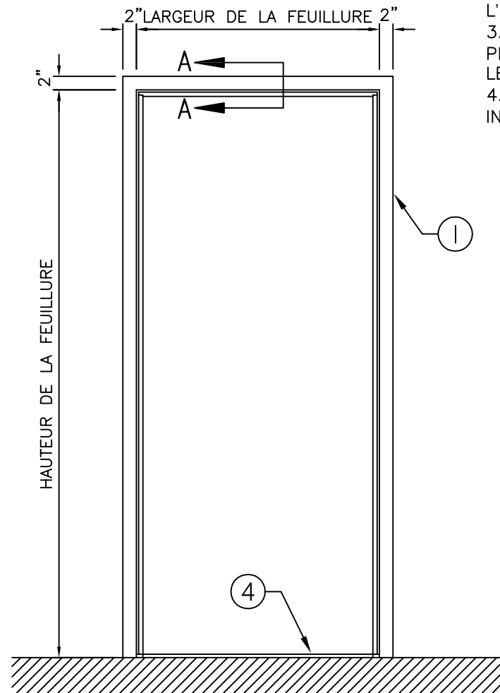
ÉLEVATION
