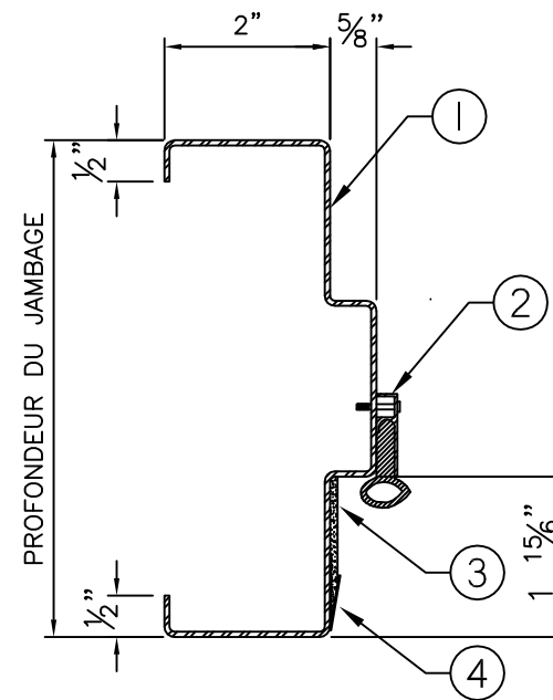
COUPE DE JAMBAGE TYPE
