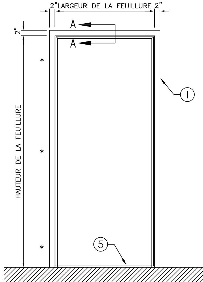
ÉLEVATION
