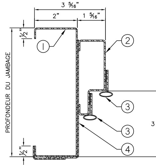
COUPE A-A
