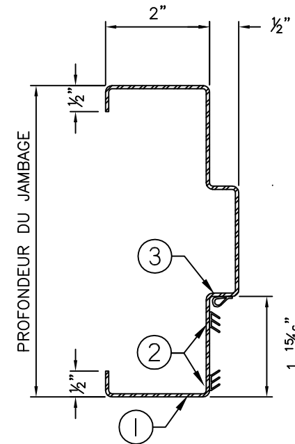
COUPE DE JAMBAGE TYPE
