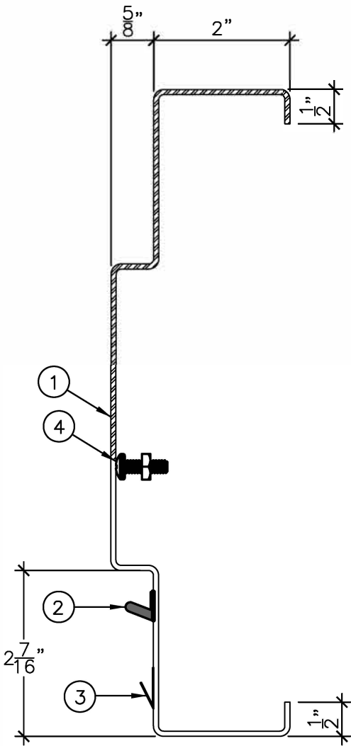
JAMB SECTION
