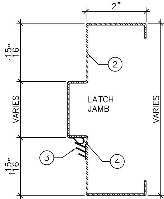
DETAIL "C" 6'' = 1'-0''
