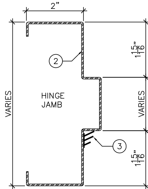
DETAIL "B" 6'' = 1'-0''
