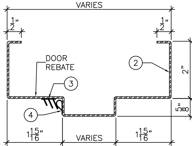
DETAIL "A" 6'' = 1'-0''
