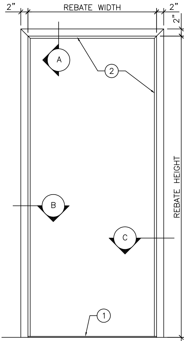
ELEVATION \frac{3}{4}'' = 1'-0''
