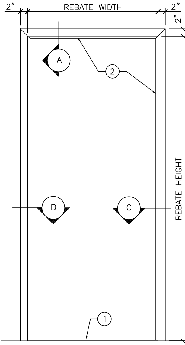
ELEVATION
