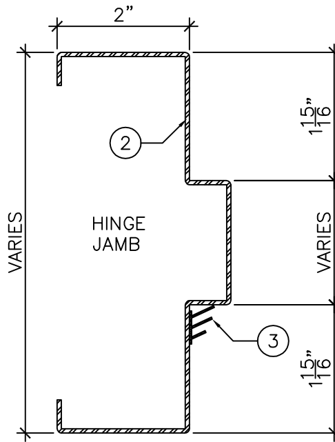
DETAIL "B" 6'' = 1'-0''
