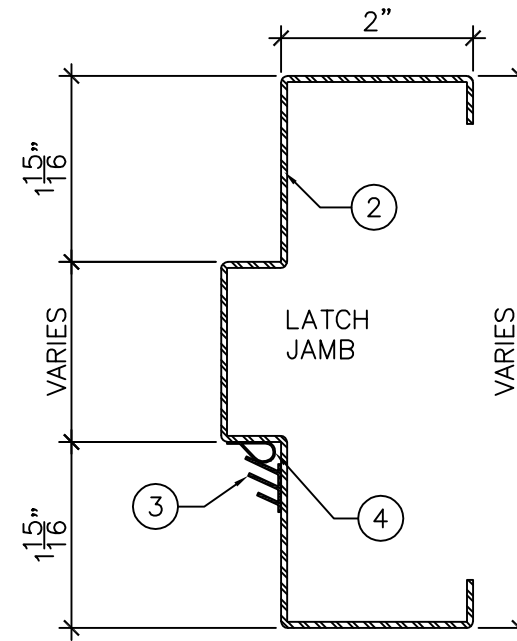
DETAIL "C" 6'' = 1'-0''
