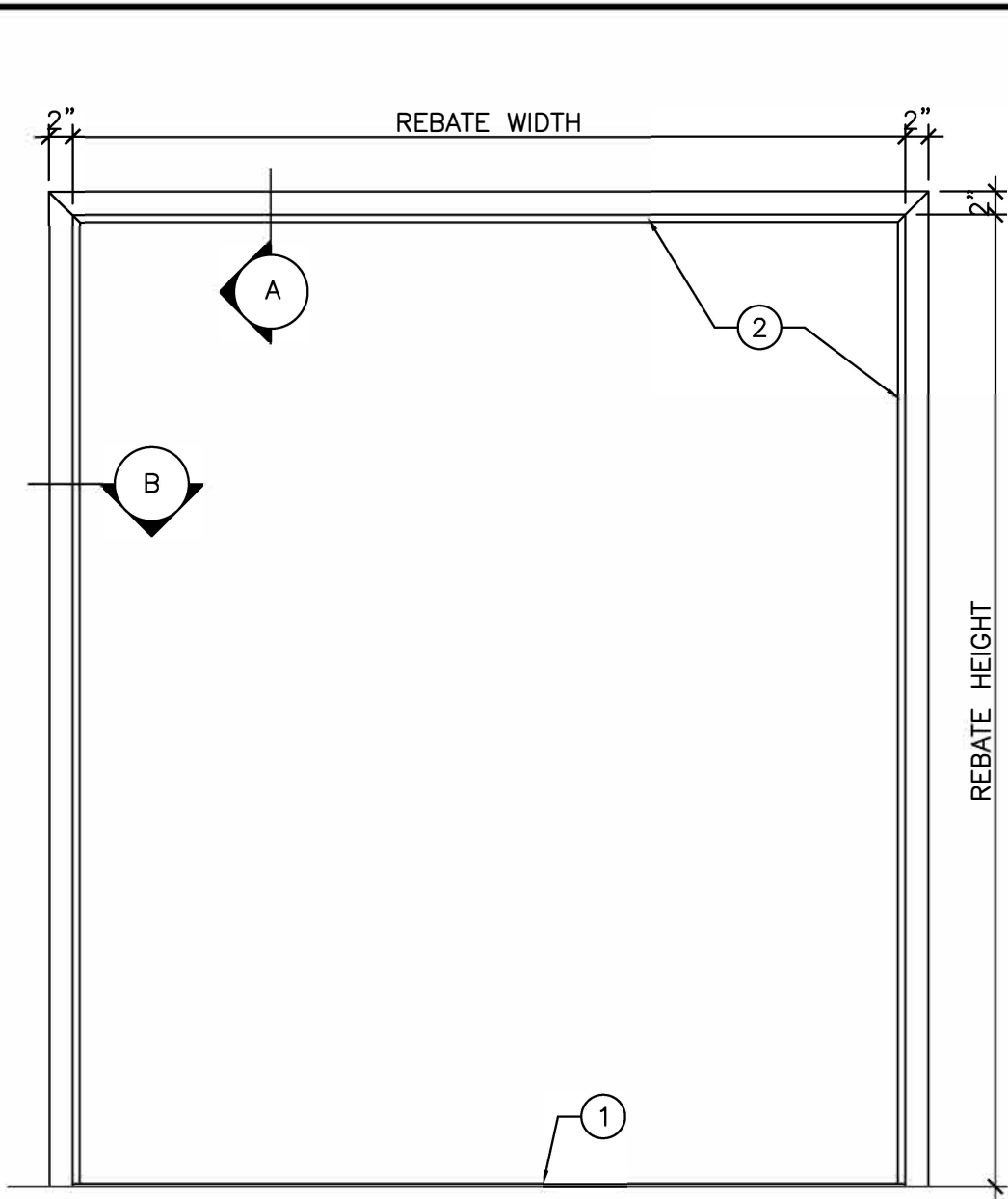
ELEVATION \frac{3}{4}'' = 1'-0''
